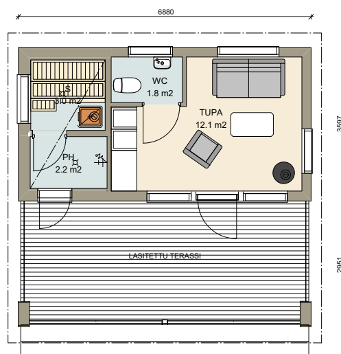
tupa, sauna, wc
