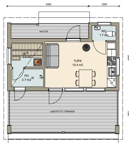
tupa, sauna, wc
