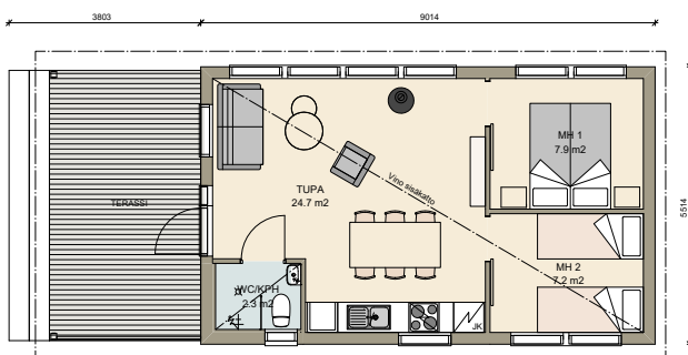
tupa, 2 mh, wc
