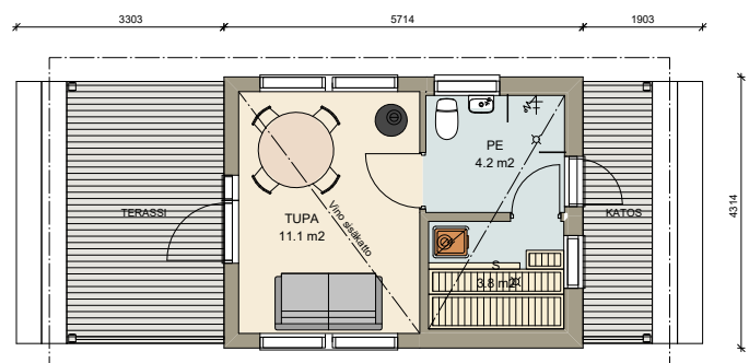
tupaa, sauna, wc
