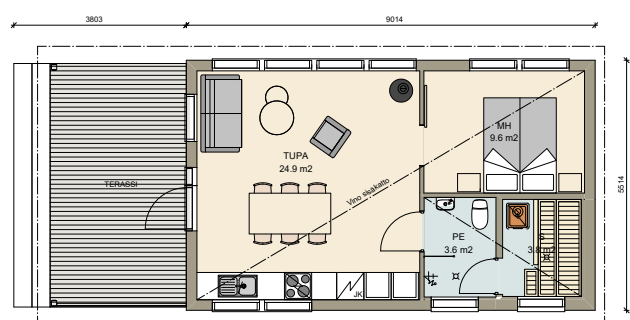
tupaa, 1 mh, sauna, wc
